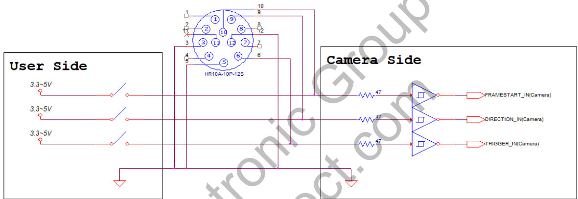
그림 7-4 Input Schematic
