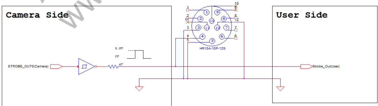
그림 7-5 Output Schematic
