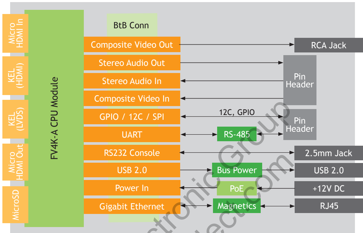
FV4K-13A Encoder
