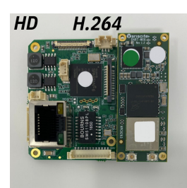
HD H.264 Aegis H.264-RM
