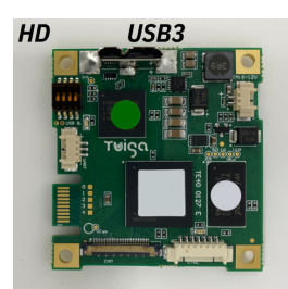
HD USB3 Aegis USB3-EV-60
